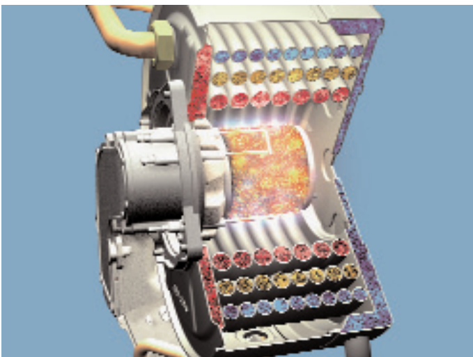
Patentierter Wärmetauscher.
